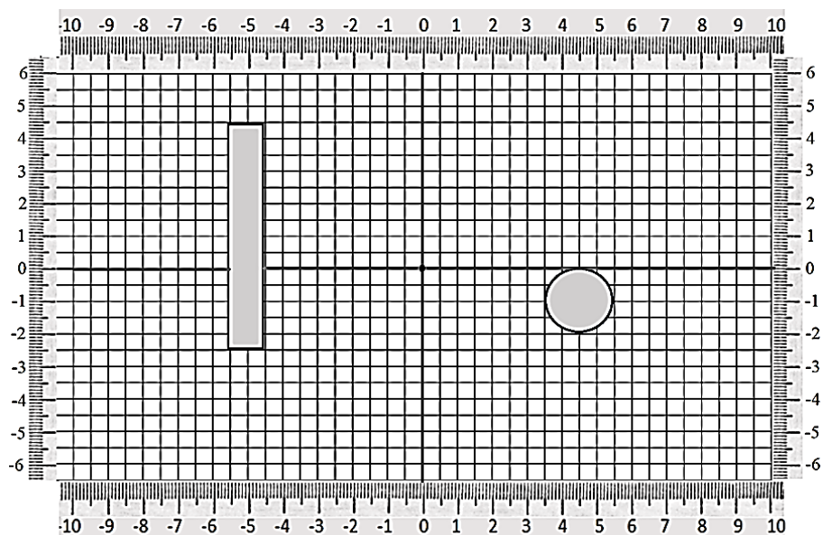
Рис.6. Координатная сетка несимметрично расположенных плоского и круглого электродов
