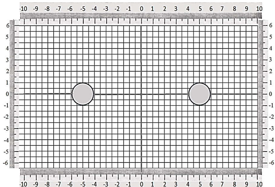
Рис.5. Координатная сетка двух круглых электродов
