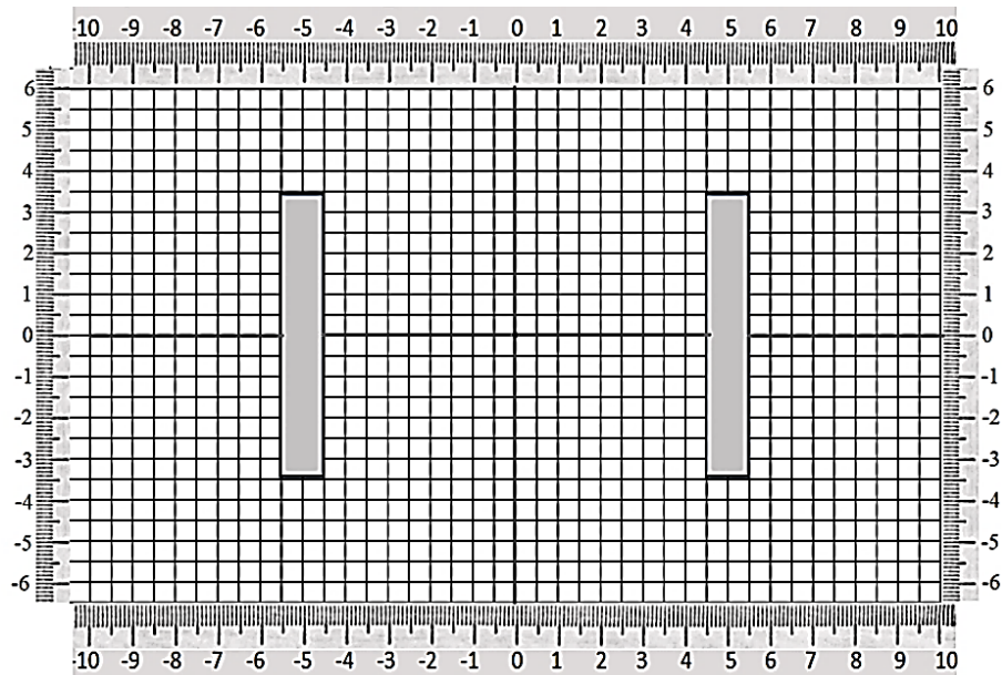
Рис.4. Координатная сетка двух плоских электродов
