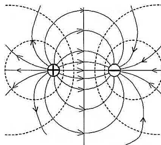
Рис.2. Пример построения силовых линий
