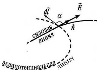
Рис.1. Экипотенциальные и силовые линии электростатического поля
